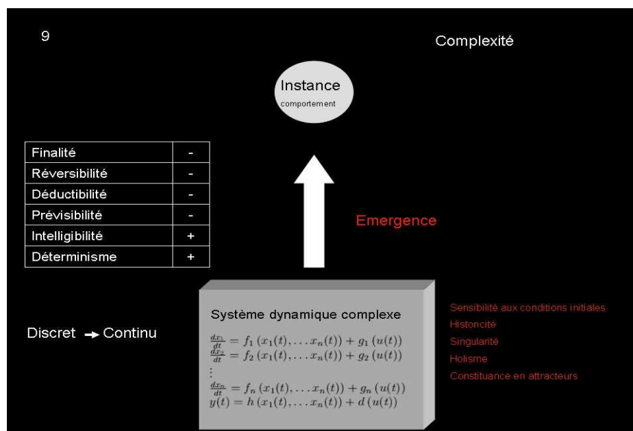
Figure 9 – Schéma type des modèles dynamiques complexes avec l'émergence d'une instance à partir d'un système dynamique complexe modélisable par des équations différentielles.
