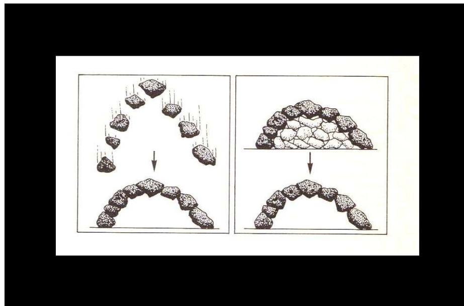
Figure 11 – 1 La probabilité pour une organisation spontanée de molécules est faible (gauche). L'organisation moléculaire a été modelée par un étayage argileux qui a ensuite disparu (droite). Tiré du livre Aux origines de la vie sous la direction de Marcel V. Locquin, p.31
